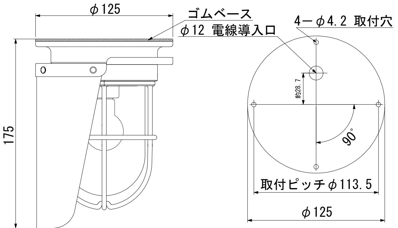
《《取付面 寸法図》》
