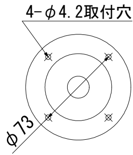
<<取付面 寸法図>>
