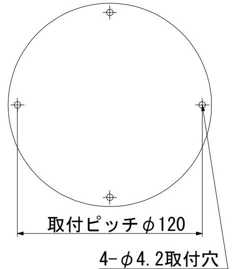
<<取付面 寸法図>>
