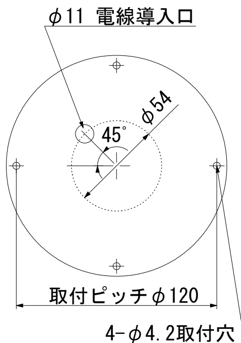
<<取付面 寸法図>>
