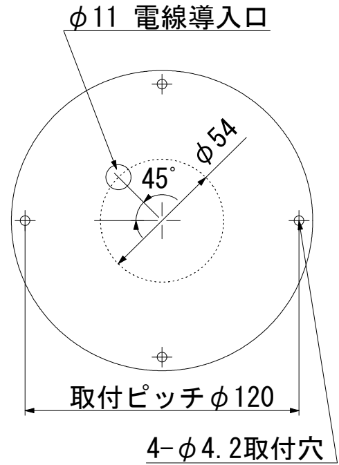
<<取付面 寸法図>>
