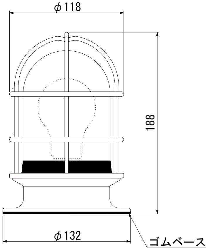
<<取付面 寸法図>>
